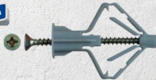
Дюбель "бабочка"+шуруп GKW
